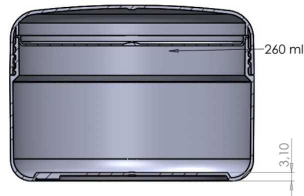
SECTION G-G SCALE 1 : 1
